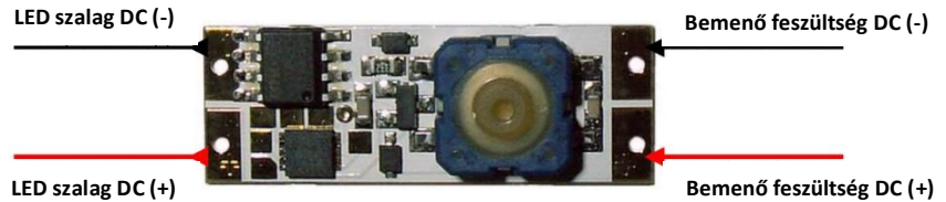
1. Kép – A fényerőszabályozó modul kimeneti csatlakozásai
