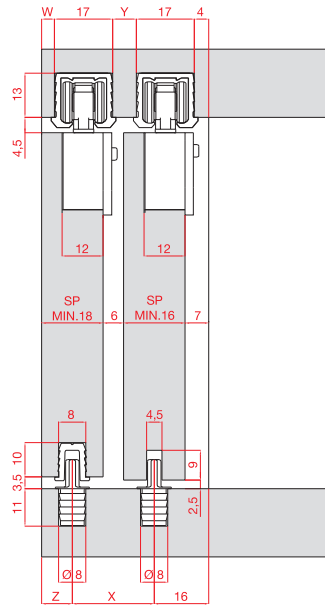
N.2 DOORS WITH SINGLE TRACK ART. 2175 / N.2 ANTE CON BINARIO SINGOLO ART. 2175
