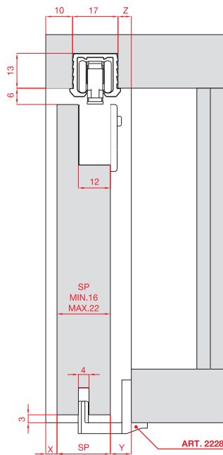
N.2 DOORS WITH SINGLE TRACK ART. 2175 / N.2 ANTE CON BINARIO SINGOLO ART. 2175
