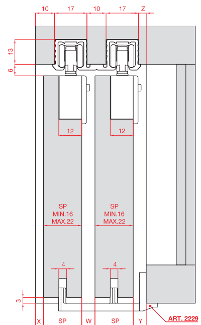
N.2 DOORS WITH SINGLE TRACK ART. 2175 / N.2 ANTE CON BINARIO SINGOLO ART. 2175
